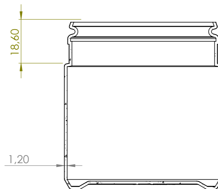
ŘEZ A-A
